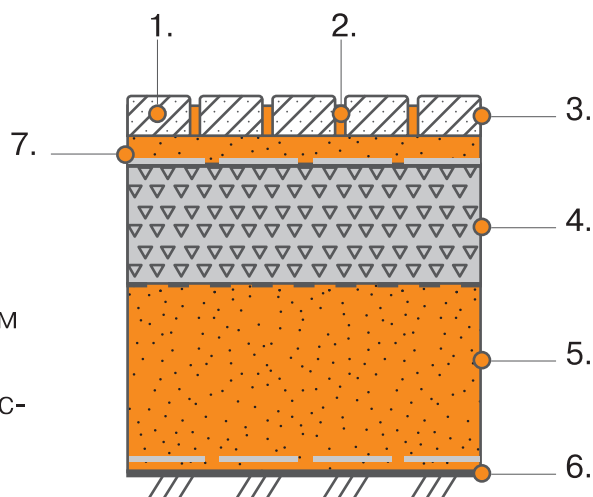
Рисунок 9. Принципиальная схема дорожной одежды с покрытием из плит бетонных тротуарных.
