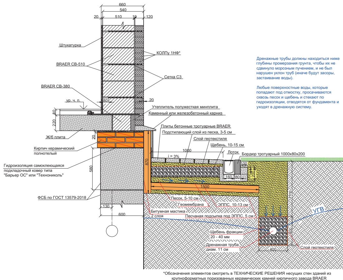
Рисунок 37. Конструкция отмонок нежесткого типа с водоотводным лотком, дренажной системой и теплоизоляцией.
