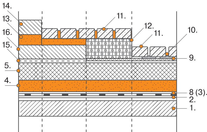
Инверсионные кровли
