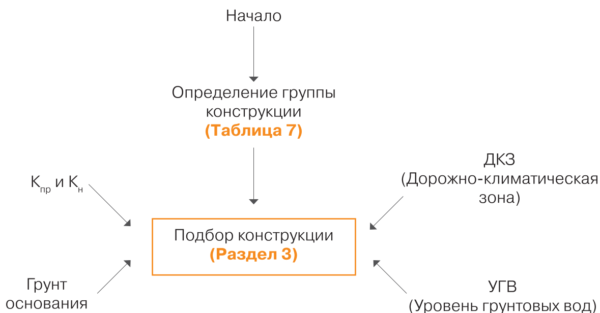
Рисунок 2. Блок-схема по использованию альбома технических решений
