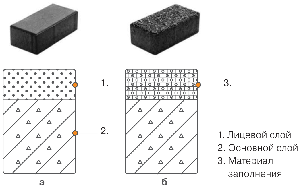
Рисунок 4. Общий вид и поперечный разрез плит бетонных тротуарных с гладкой (а) и размытой (фактурной) лицевой поверхности (б)
