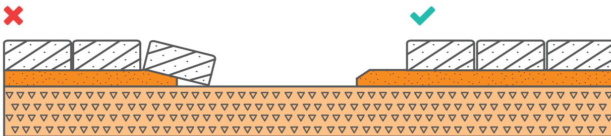
Рисунок 39. Неправильный и правильный варианты ремонта покрытия
