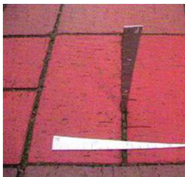
Рисунок 40. Измерение ширины шва при восстановлении покрытия
