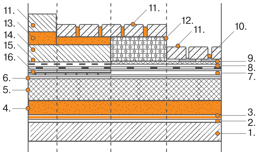
Эксплуатируемые кровли
