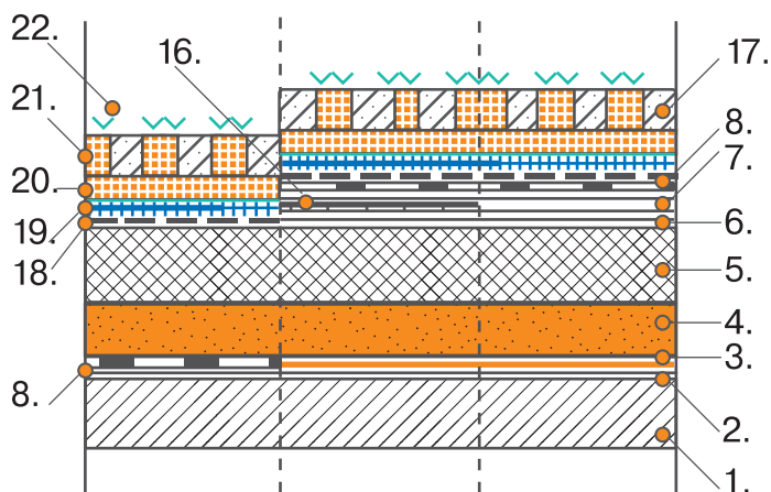
Озелененные кровли
