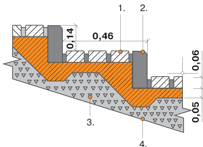
Рисунок 17. Вариант устройства лестниц
