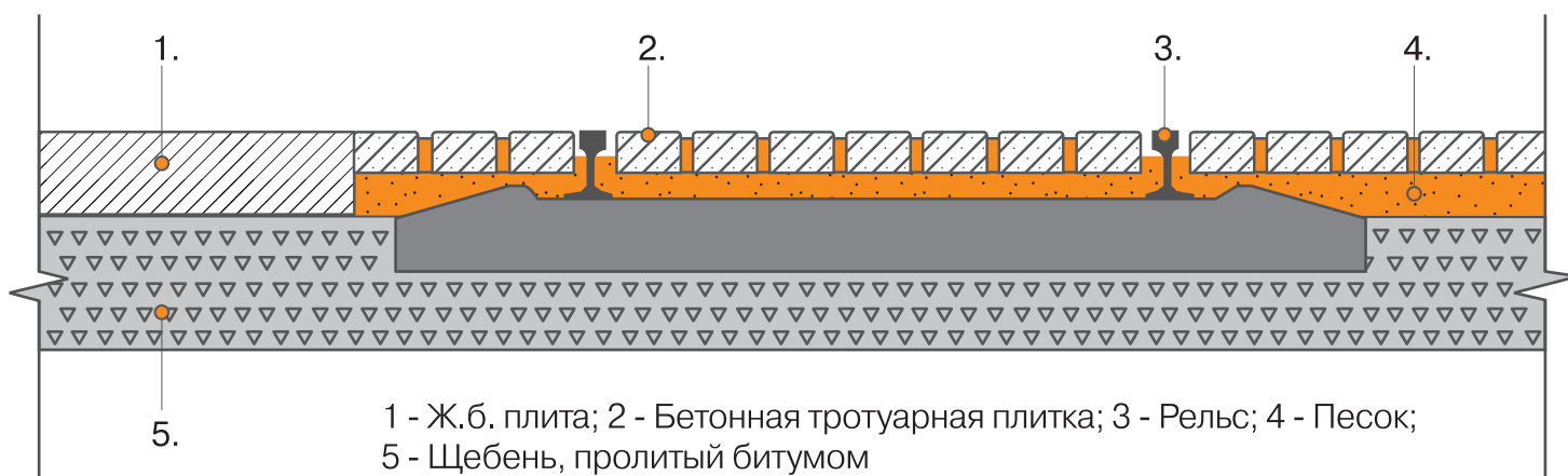
Рисунок 22. Конструктивная схема трамвайных путей с покрытием из плит бетонных тротуарных Группы VI
