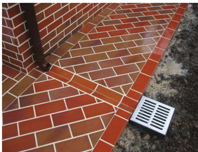
Рисунок 38. Сброс воды с крыши в ливневую канализацию.
