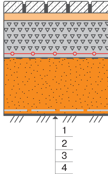
Рисунок 23. Конструктивная схема дорожной одежды с покрытием из плит бетонных тротуарных BRAER Группы ВII
