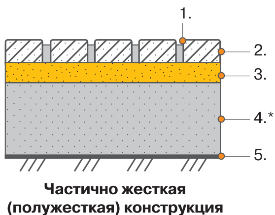
Рисунок 10. Схемы конструкций дорожных покрытий с несвязанными покрытиями.
